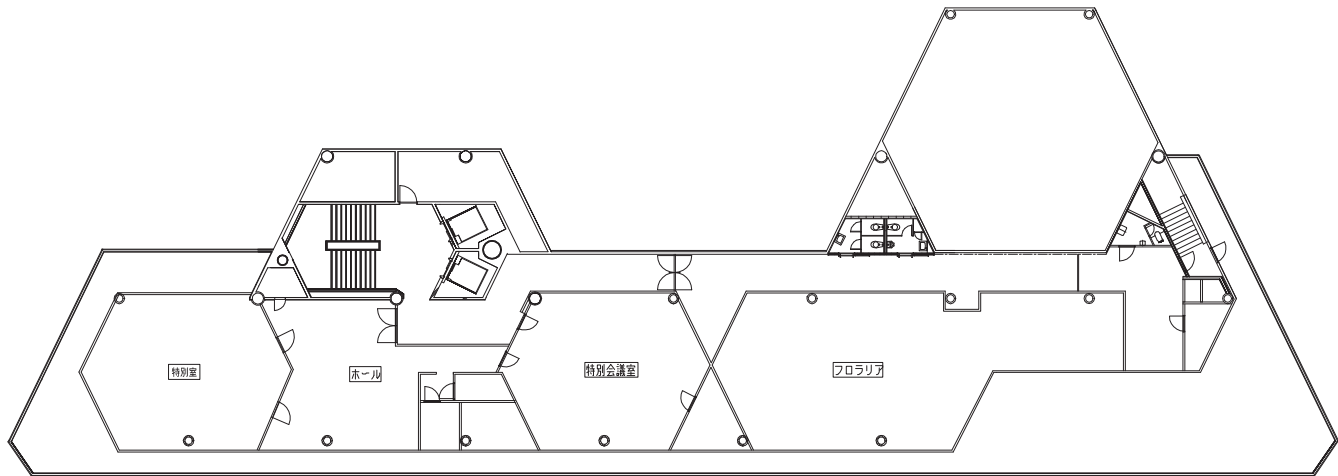
6階平面図
