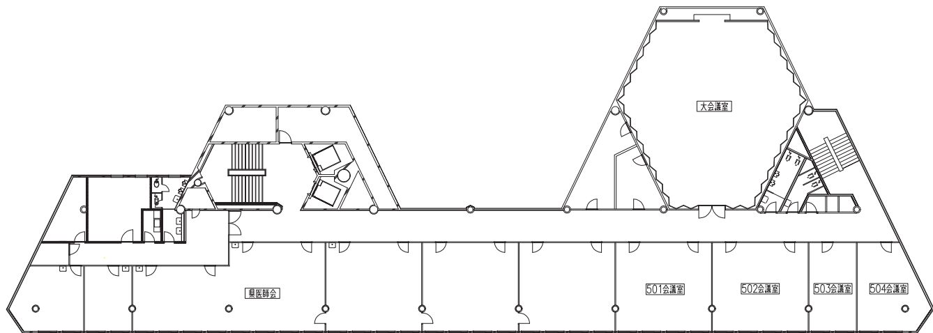
5階平面図
