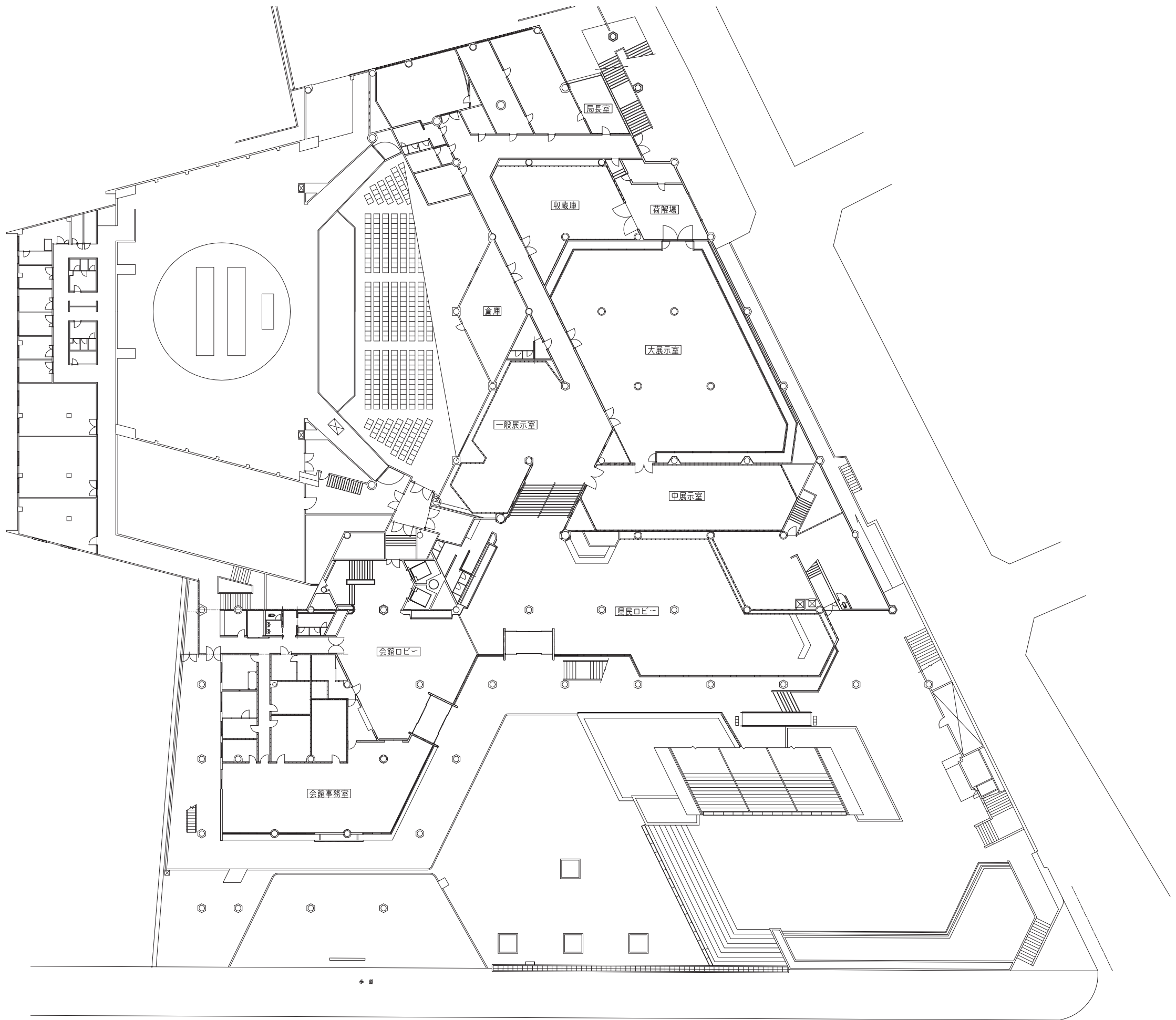
1階平面図
